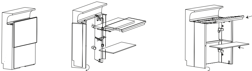
Modulo chiuso Closed element Aprire le due ante e inserire il piano Open the two sides and place the top
