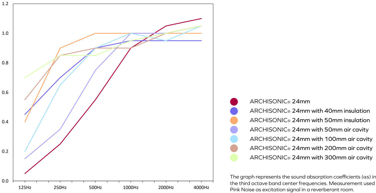
Sound Absorption Coefficient (α s ) according to EN ISO 354 Universität Stuttgart – Institut für Akustik und Bauphysik IABP
