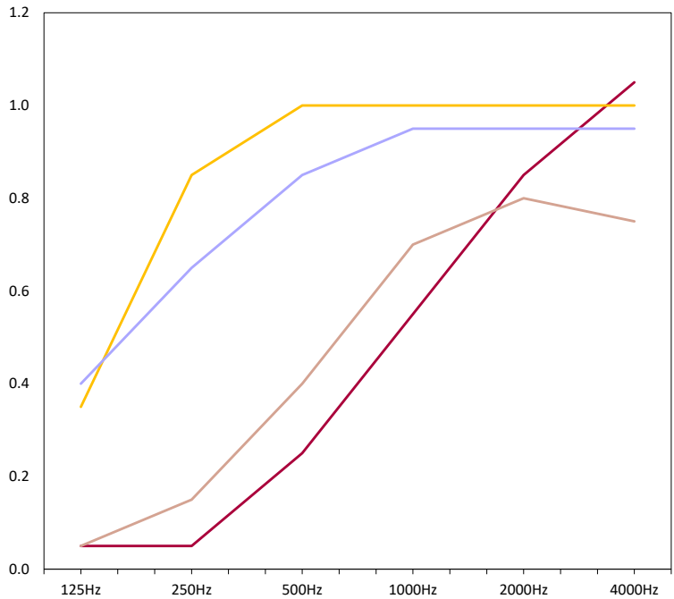
Sound Absorption Coefficient ( \alpha_s ) according to EN ISO 354 Universität Stuttgart – Institut für Akustik und Bauphysik IABP
